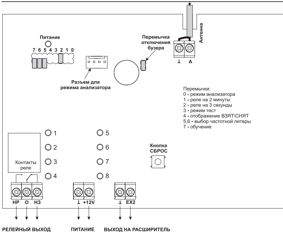
Рис. 4. Монтажная схема приёмника
