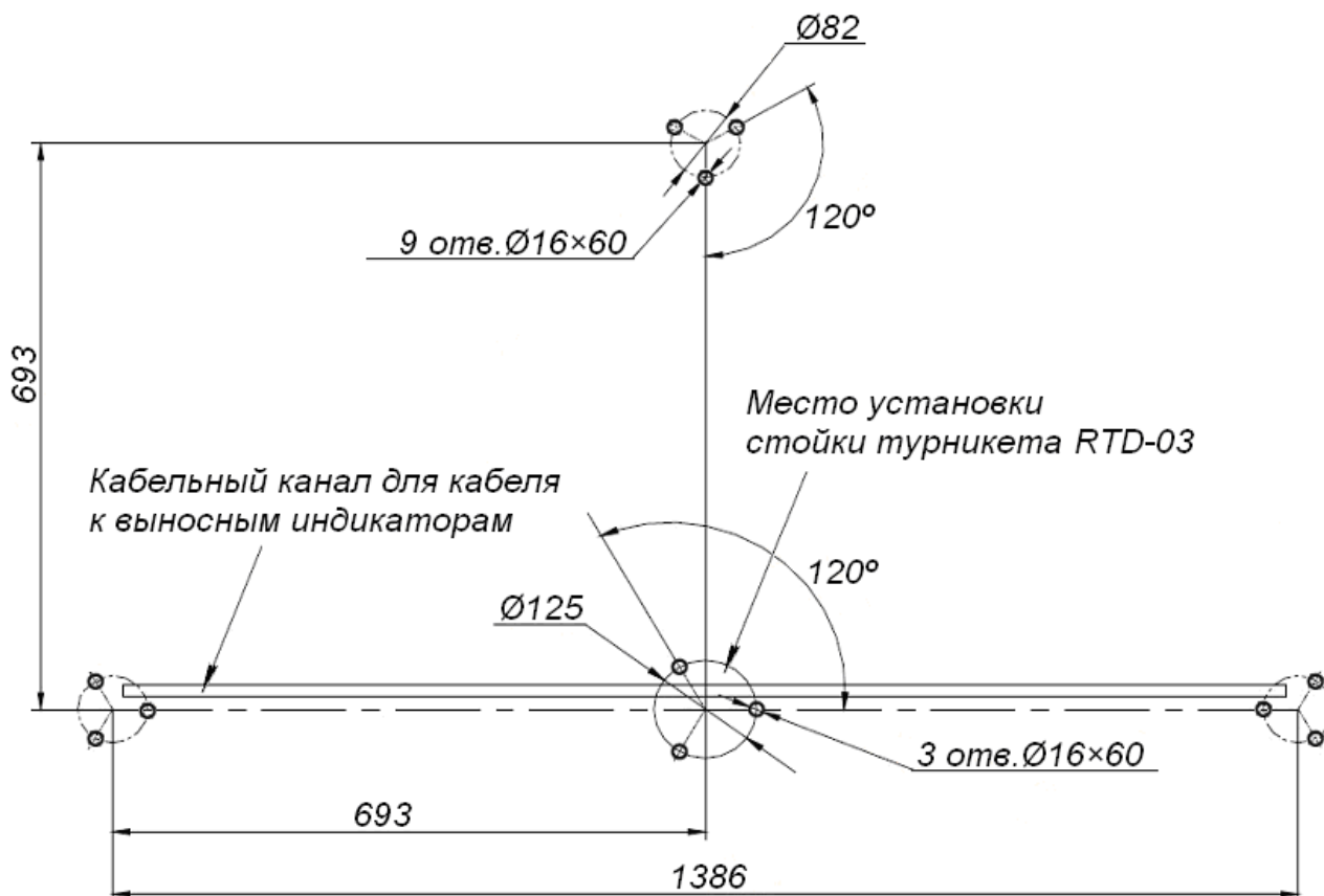
Рисунок 14. Схема разметки для монтажа турникета с формирователем прохода (кабельный канал к блоку управления прокладывается от центра стойки турникета в направлении БУ в соответствии с планировкой)
