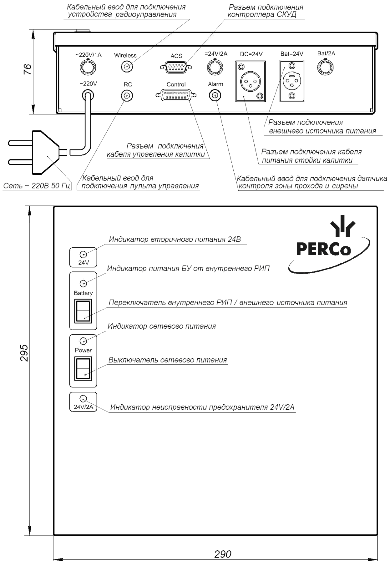
Рисунок 5. Блок управления
