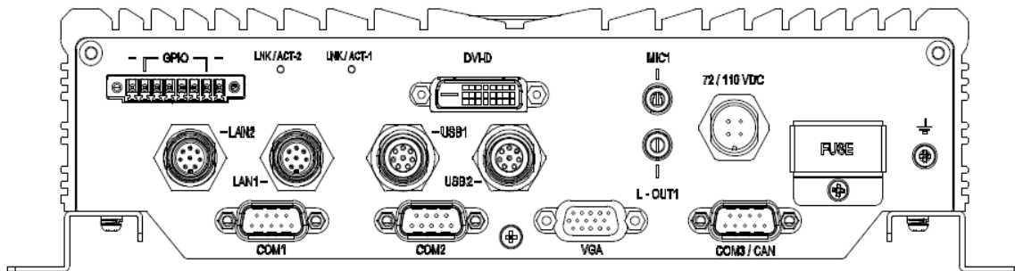
Вид спереди
