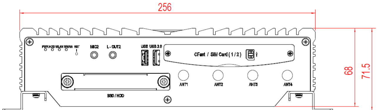
Вид сзади
