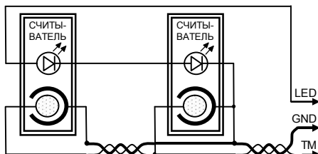
а) подключение «цепочкой»
