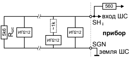
б) токопотребляющие датчики
