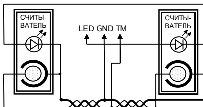
б) подключение «звездой»
