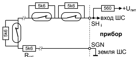
а) нормально замкнутые датчики
