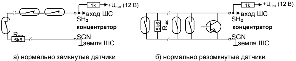
Рисунок 7 – Примеры монтажа охранных шлейфов
