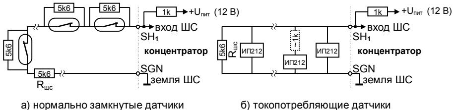
Рисунок 8 – Примеры монтажа пожарных шлейфов
