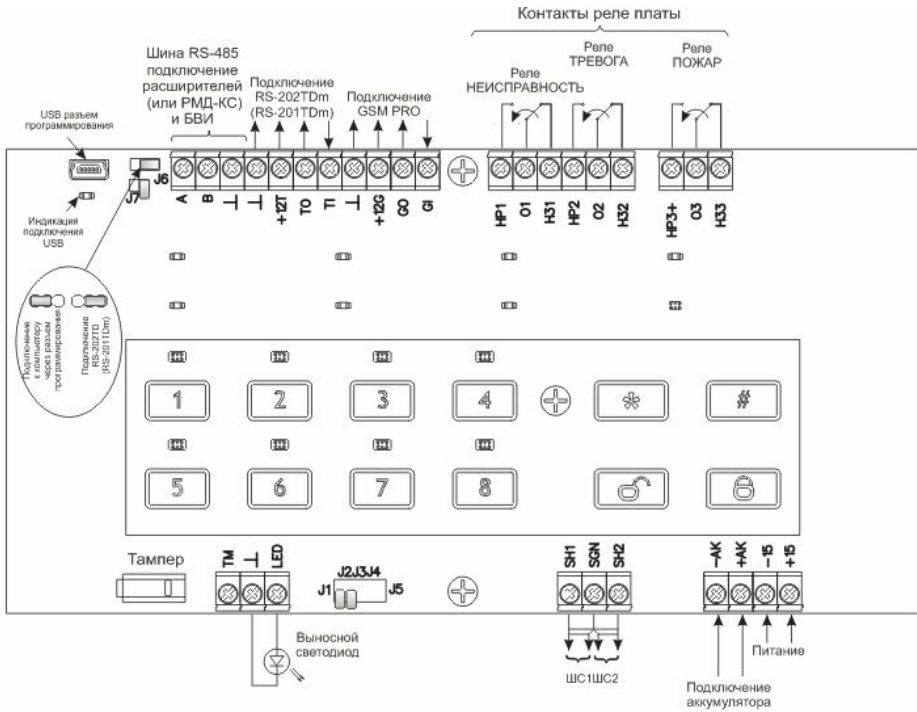
Рисунок 11 – Монтажная схема концентратора
