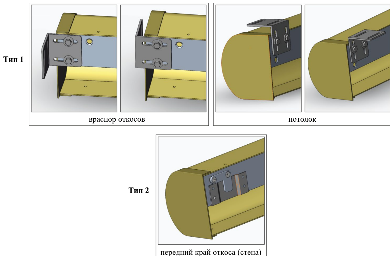
Рисунок 3 – Типы крепления ВШ
