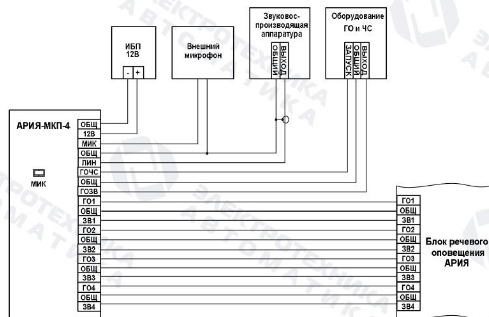
Рис.1. Схема подключения.
