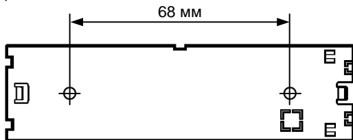
Рис.9 Присоединительные размеры
