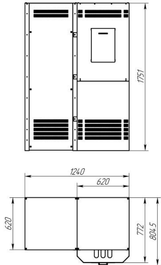
Сборка стеллажа CA-20-250 (M) с секцией на широкой стороне
