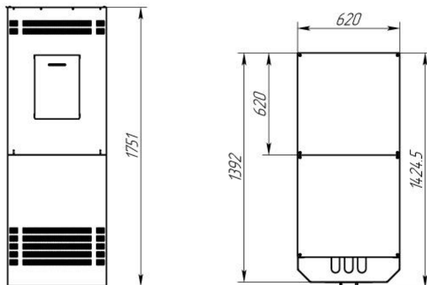
Сборка стеллажа CA-20-250 (M) с секцией на узкой стороне
