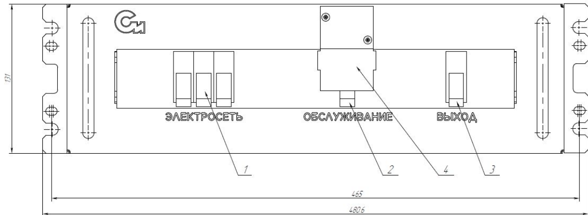
Рис. 1. Габаритно-присоединительные размеры ББ. Вид спереди.
